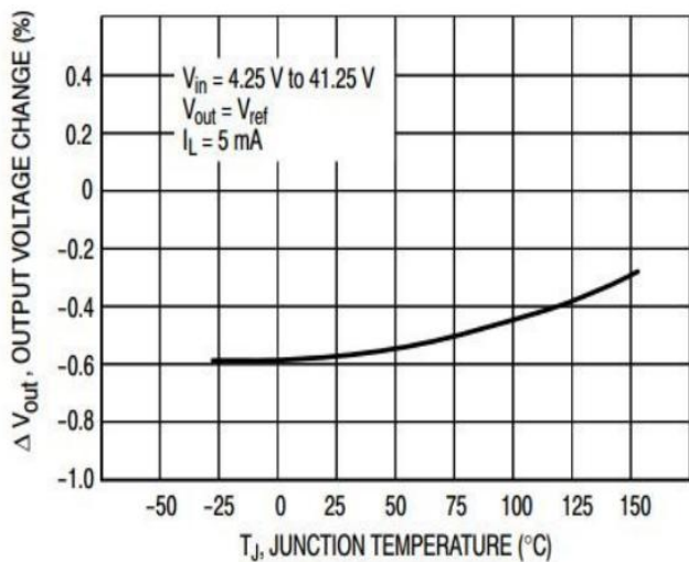
图 13 线性调节
