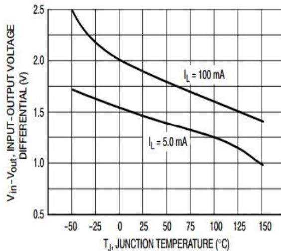
图 8 差电压
