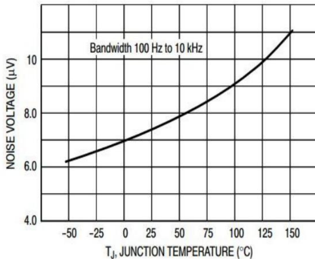
图 14 输出噪声
