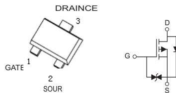
SOT-723
