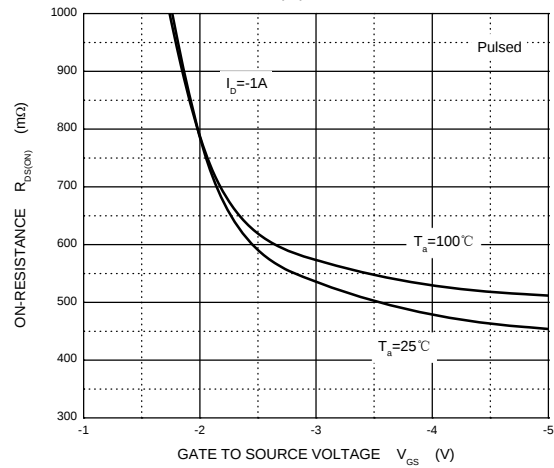
R_{DS(ON)} — V_{GS}
