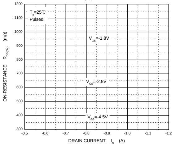
R_{DS(ON)} — I_D
