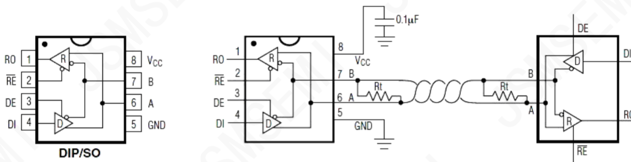
图 3: MAX13085EESA+T典型半双工应用电路
