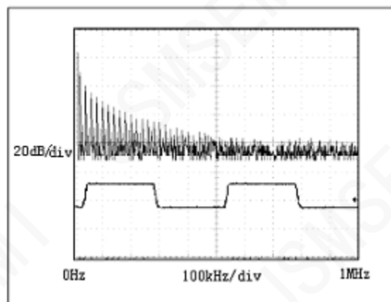
图 13: 传输 20kHz 信号时 MAX13085EESA+T 驱动器输出 波形和 FFT 图
