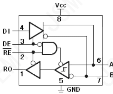
图2: MAX13085EESA+T逻辑图
