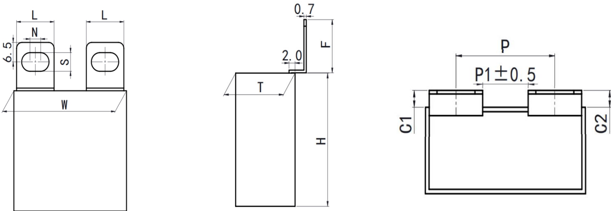
Style A Horizontal installation 水準安裝
