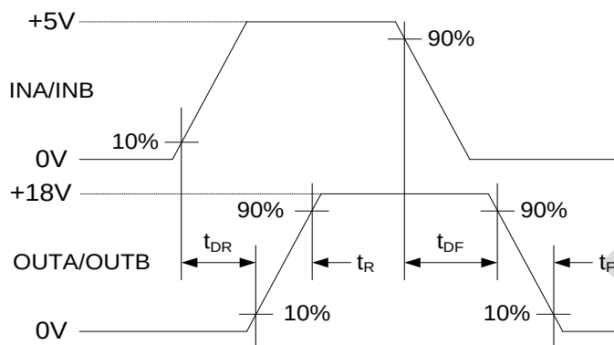
图 1 开关参数波形图
