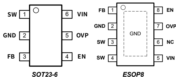
图 3.1 封装与引脚排列
