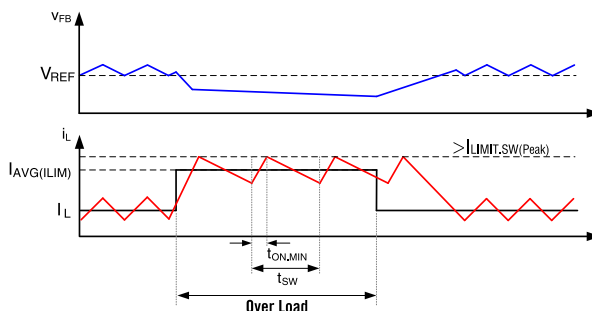
图 8.1 BUCK 输出过流于 M_{top} 行为描述
