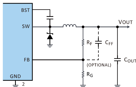
图 5.1 BUCK 恒压模式与 CFF 前置补偿电容
