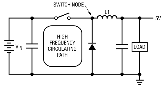
图 14.2. 高速开关通路
