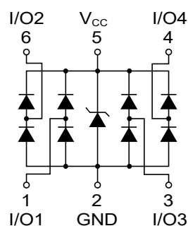
SOT23-6
