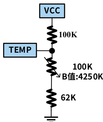
图 8.TEMP 管脚电阻配置（串联型）
