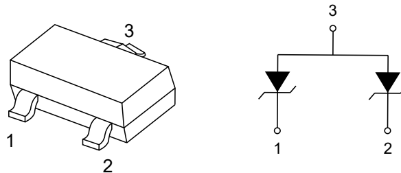
SOT-23
