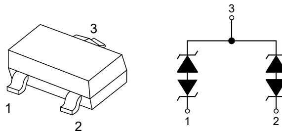
SOT-23
