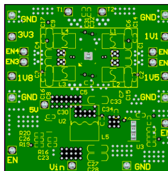
PCB GND layer
