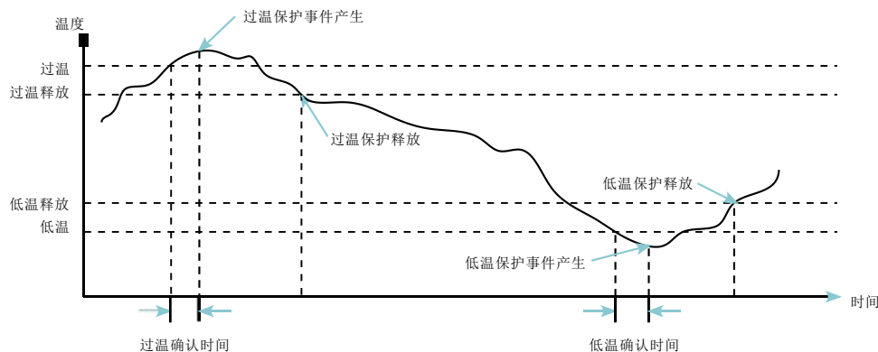
图 18: 温度保护示意图
