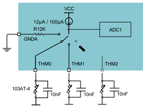
图 14：高压采集前端内部温度测量示意图
