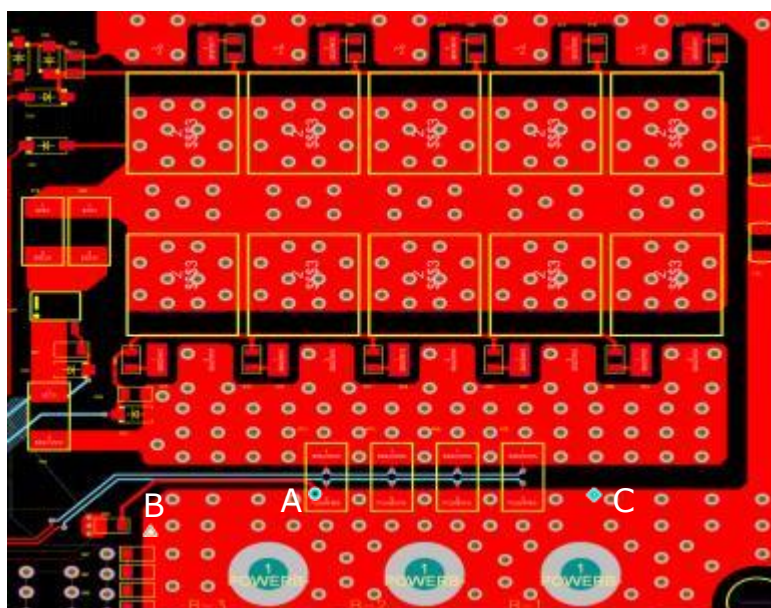
图 17: AGND 布局建议
