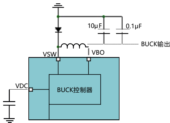
图 11: 典型高压 Buck 应用图
