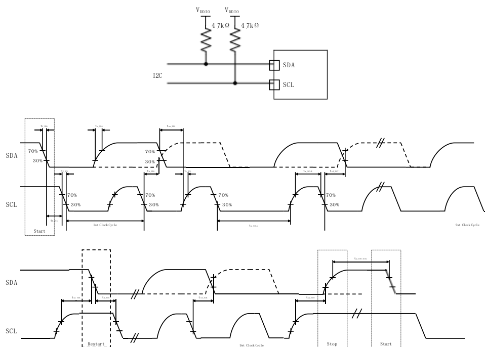
图 4: I2C 交流波形
