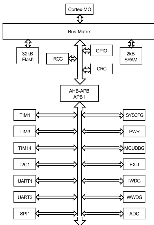
图 9: AMG8605 数字内核内部框图
