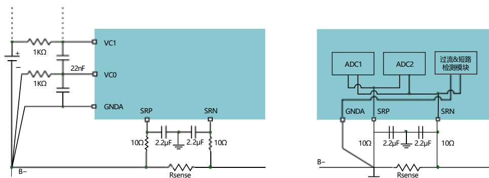
图 13: 电流采样推荐电路设计以及内部结构示意图
