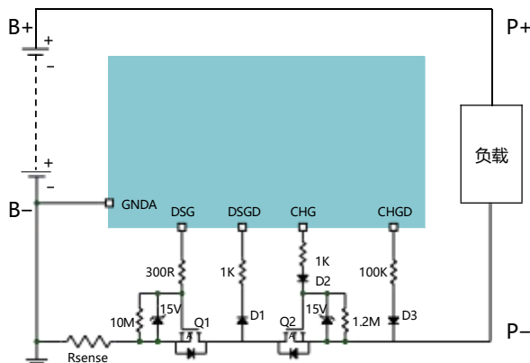
图 15: 充电器/负载检测
