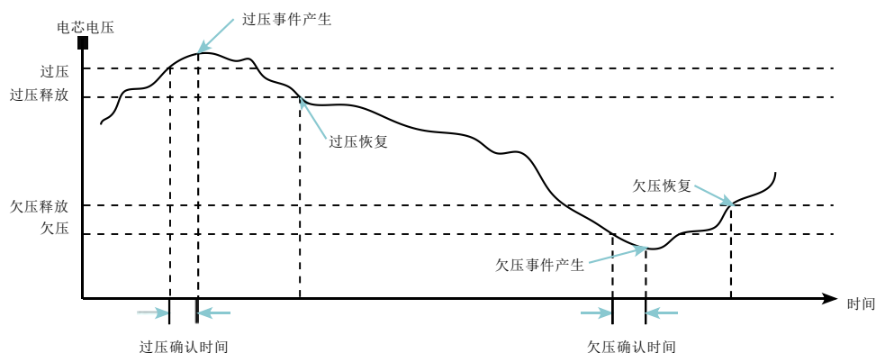
图 16: 过欠压保护示意图
