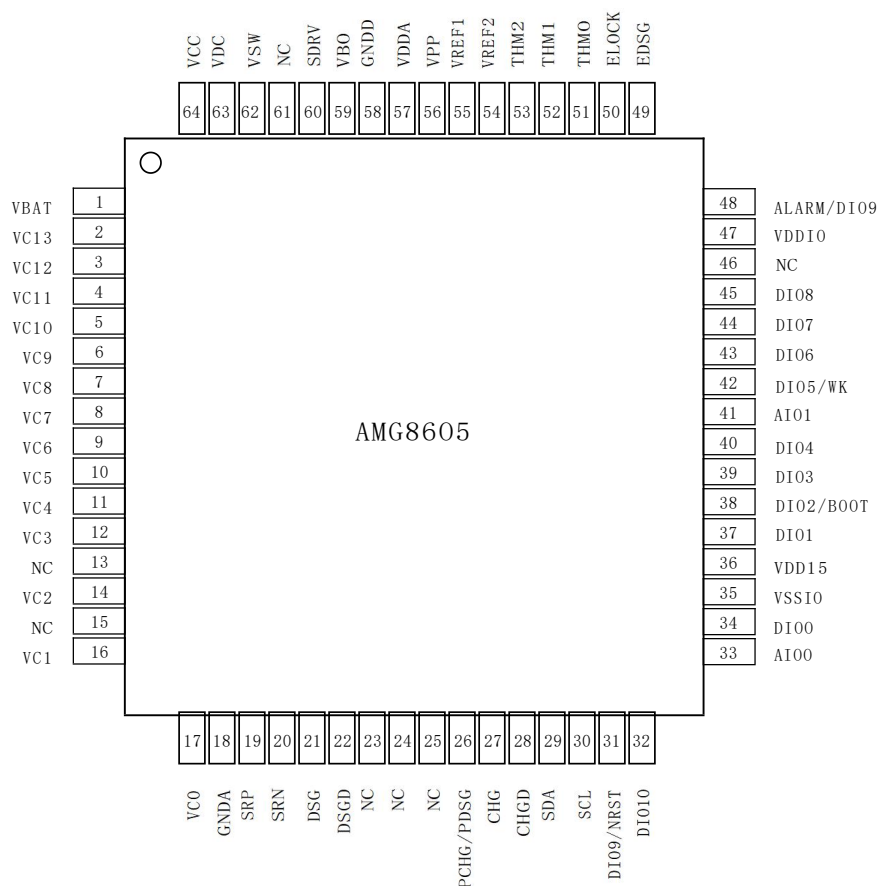
图 1: AMG8605 引脚图
