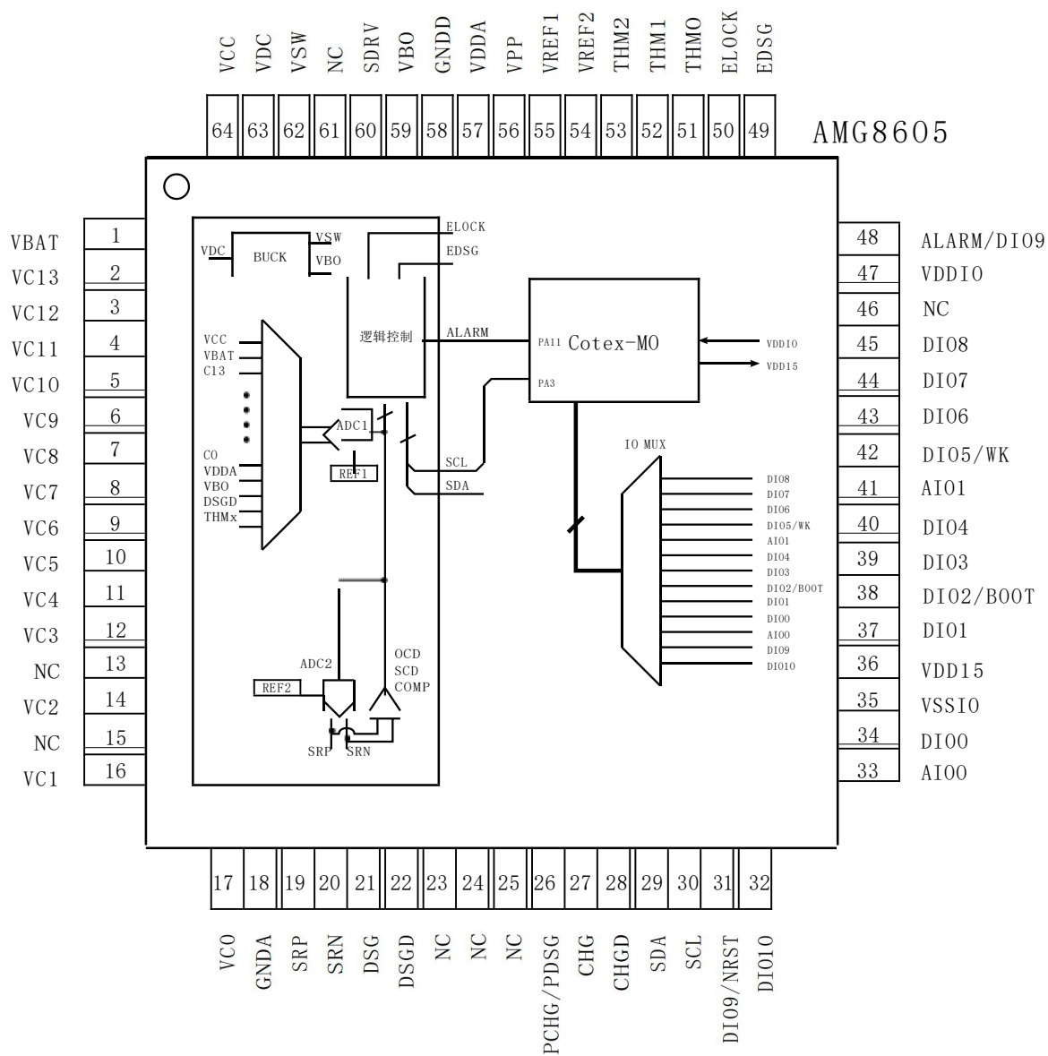
图 8: AMG8605 内部框图
