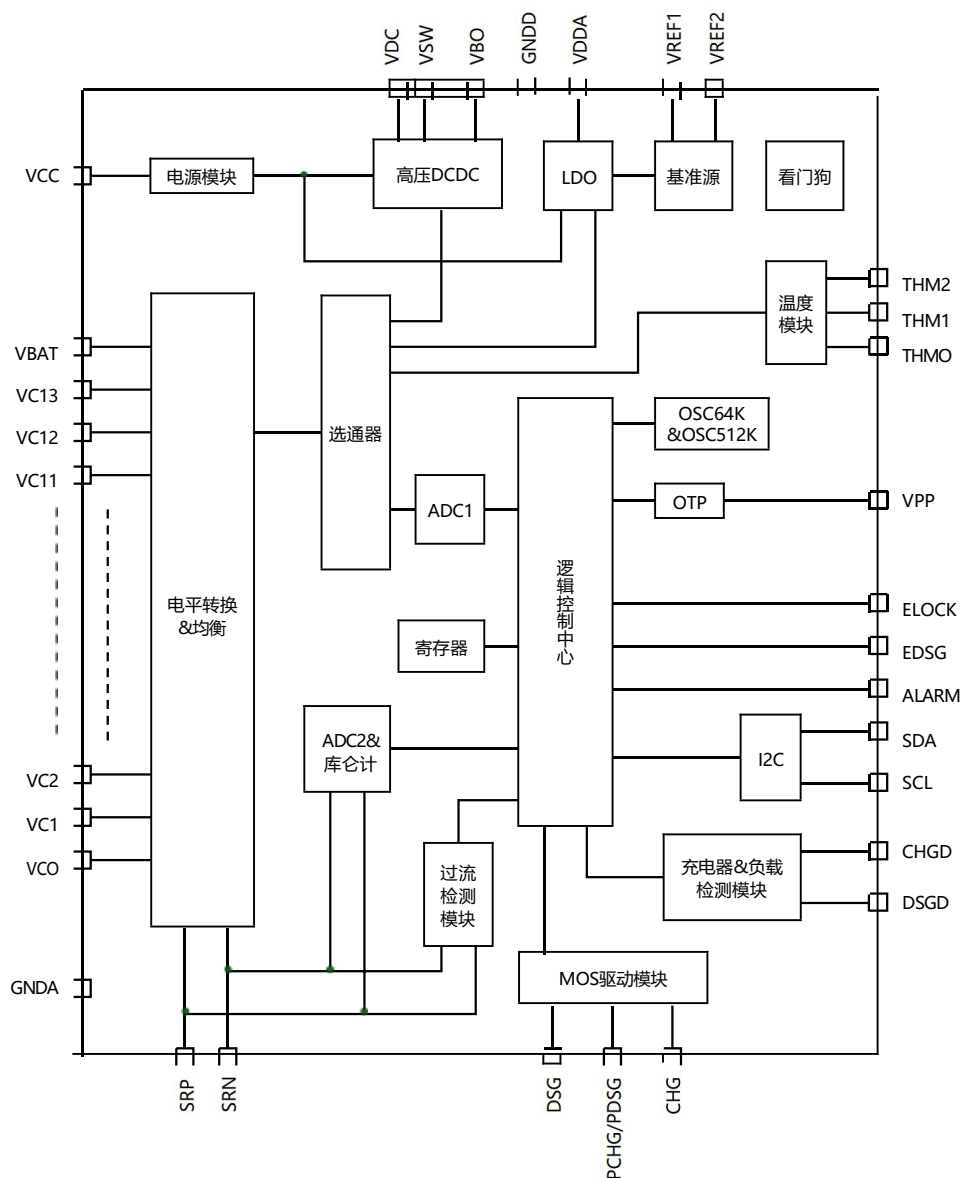
图 10: 高压采集前端内部框图
