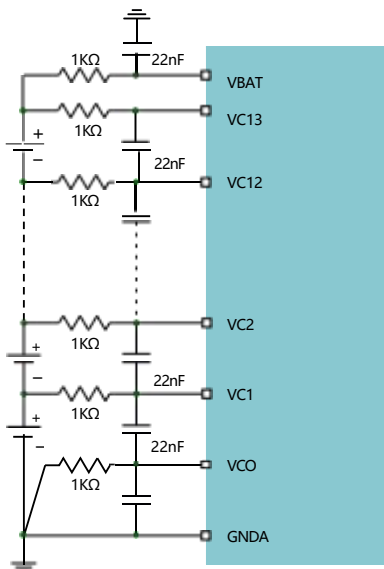
图 12: 电池电压输入滤波电路
