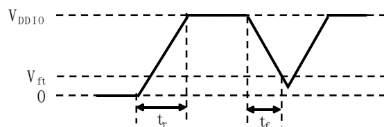
图 2: 上电时间和下电时间
