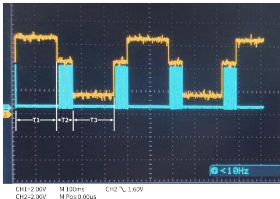
图 21: 电池自动均衡时序
