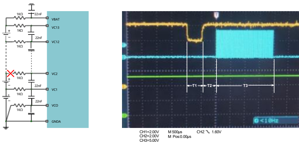
图 19: 断线诊断示意图
