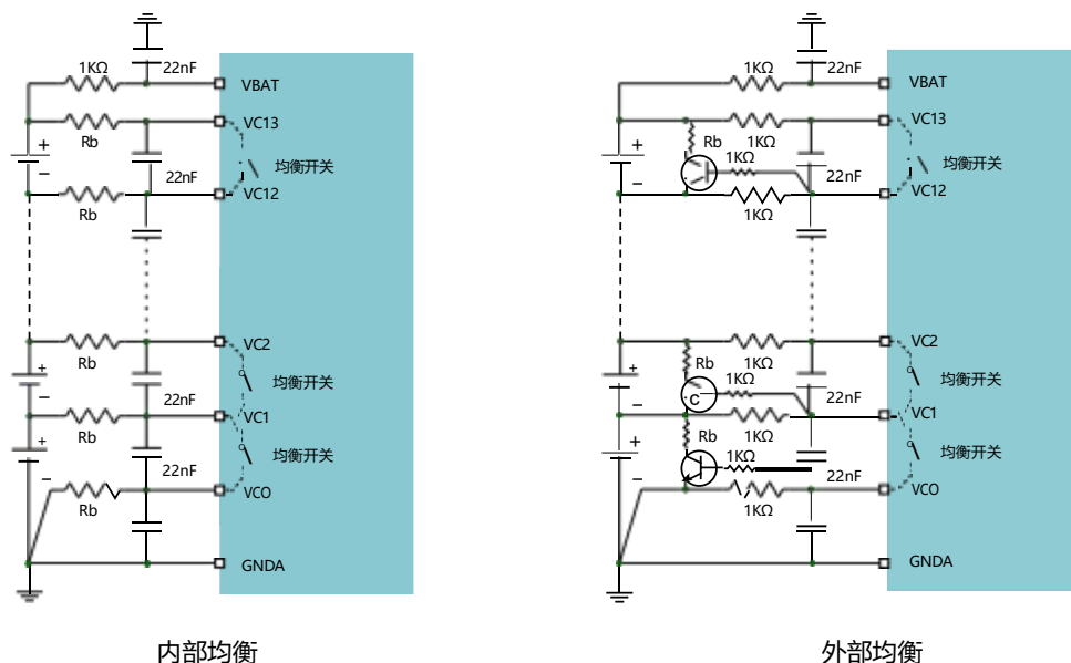
图 20: 电池被动均衡电路示意图
