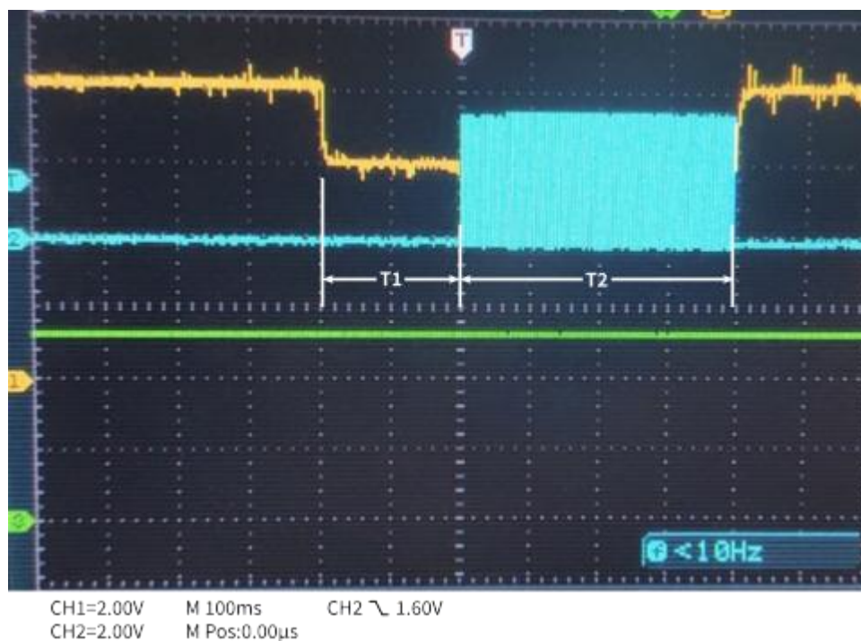
图 22: 电池手动均衡时序
