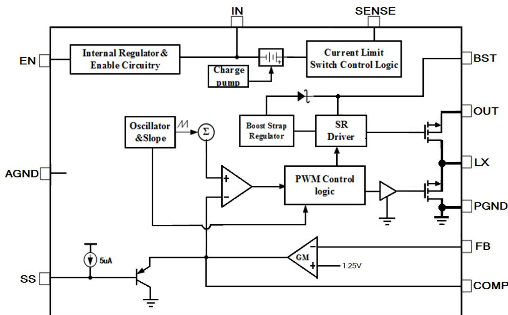
图 1: HT3080A 功能框图
