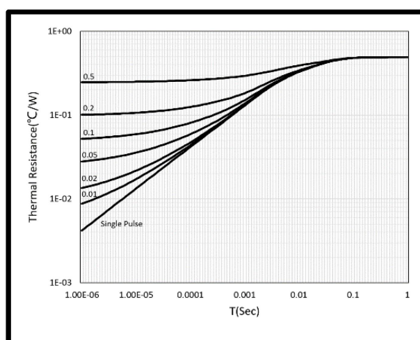
图 8 瞬态热阻抗
