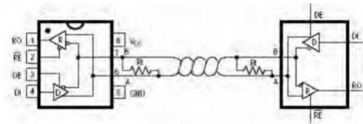
图2产品应用示意图
