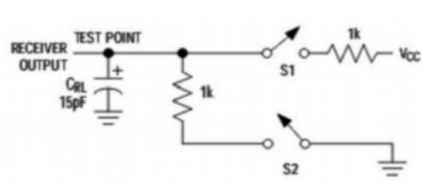
图4 接收时间测试电路
