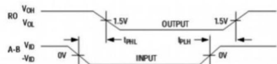
图9接收传输延时
