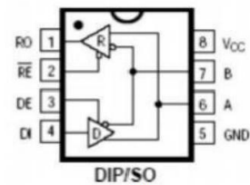
图1封装图
