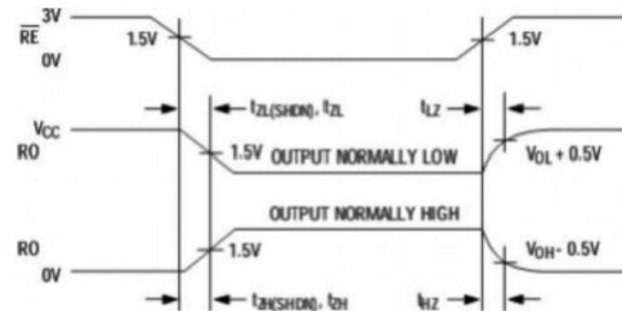
图 1 1 接收开启和关闭时间
