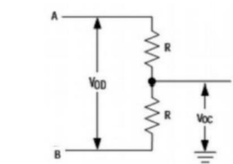
图3 直流驱动测试电路
