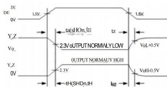
图10驱动开启和关闭时间
