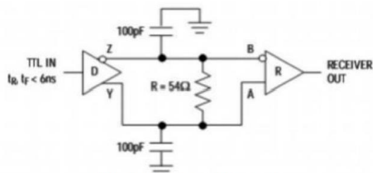
图7接收传输延时测试电路
