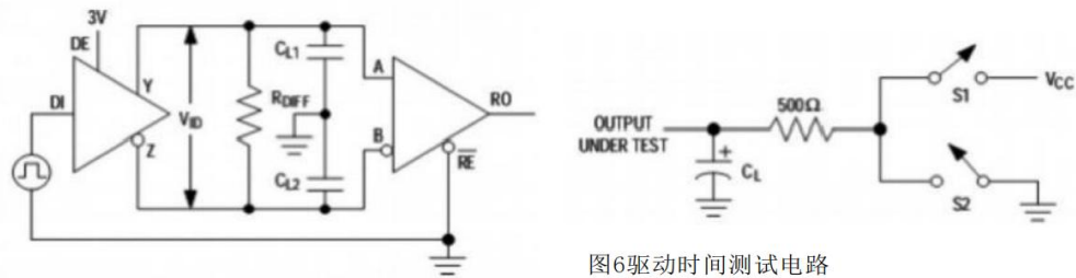
图6驱动时间测试电路
