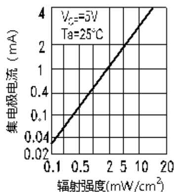
图五：集电极电流VS辐射照度
