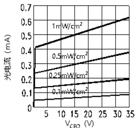
图六：光电流VS VCE曲线
