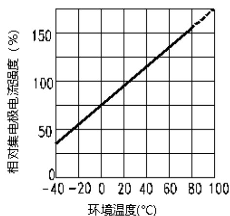
图四：相对集电极电流强度VS环境温度曲线
