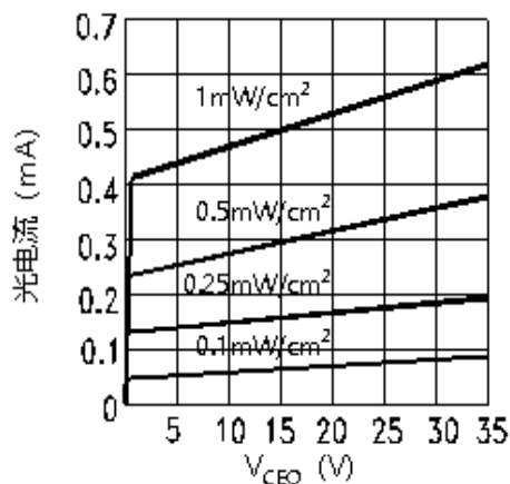
图六：光电流VS VCEO曲线
