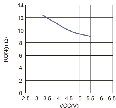
Rds_on vs.Vcc
