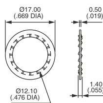
LOCKWASHER
