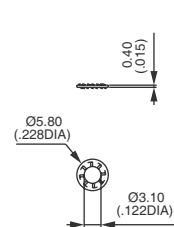
LOCKWASHER
