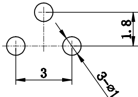
PCB线路板安装图(±0.1)
