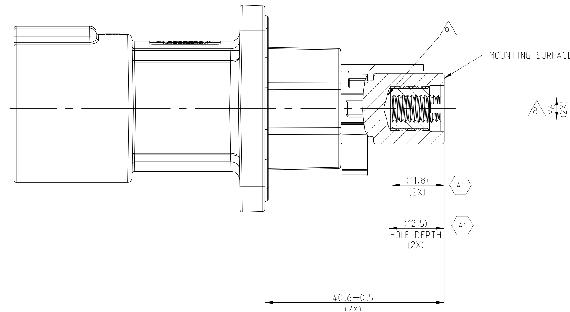
SECTION A-A
