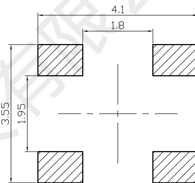
安装参考图
