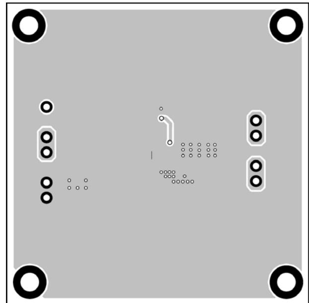
Figure 2—Bottom Layer
