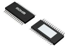
HTSSOP-B28 BD81A74EFV-M
