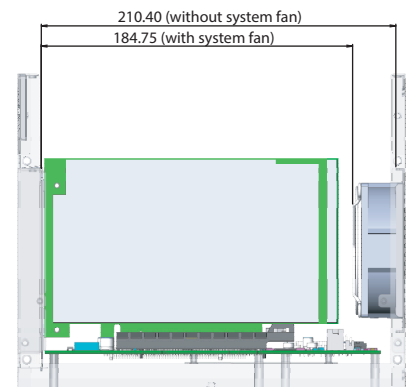
4-slot i-Module
