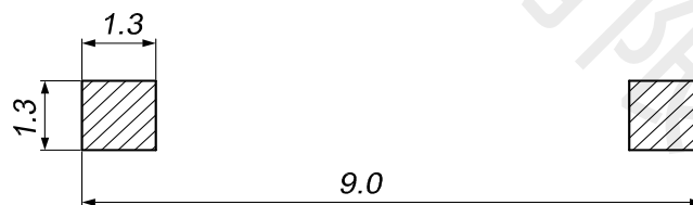
印制线路板 Recommended P.C.B layout
