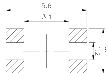
PCB. 焊接图
