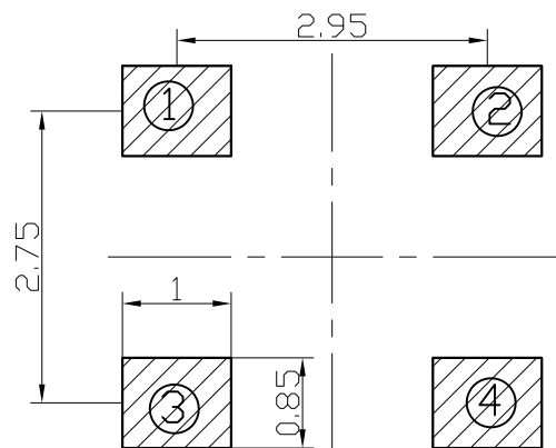
安装参考图
