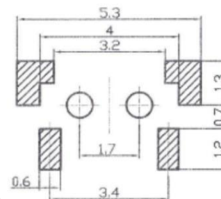
安装参考图
