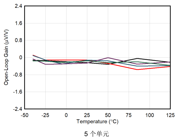
图 6-28. 开环增益与温度间的关系
