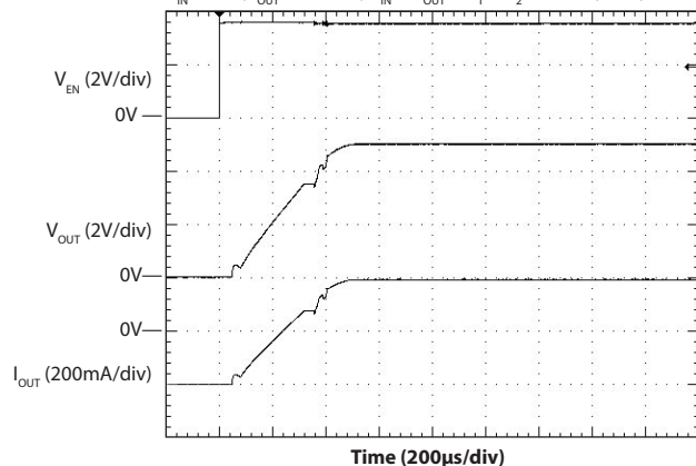
Startup (400mA)
