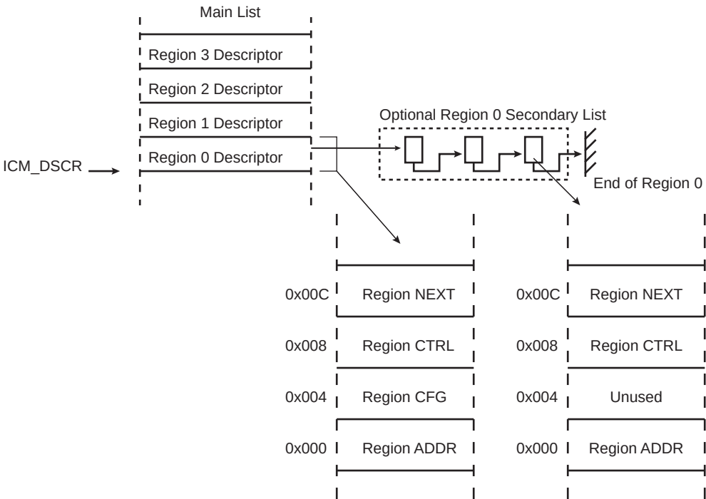
Figure 55-4. Region Descriptor
