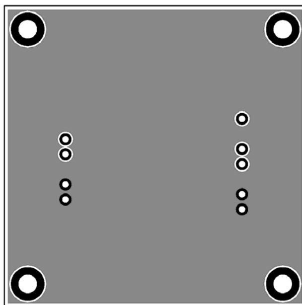
Figure 3—Bottom Layer
