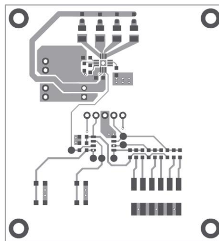
Figure 2—Top Layer
