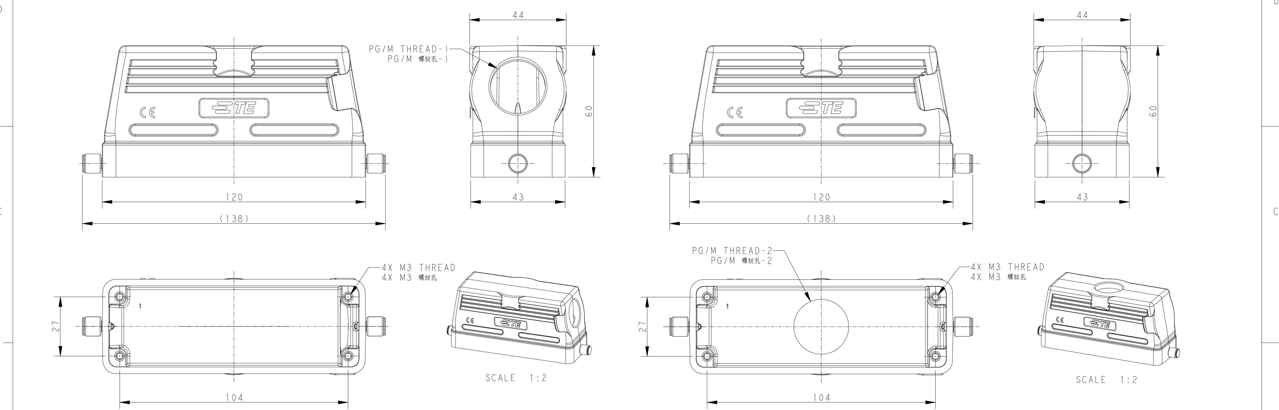
TYPE 1: LOW CONSTRUCTION, SIDE ENTRY 类型1： 低结构， 侧出 TYPE 2: LOW CONSTRUCTION, TOP ENTRY 类型2： 低结构， 高出
