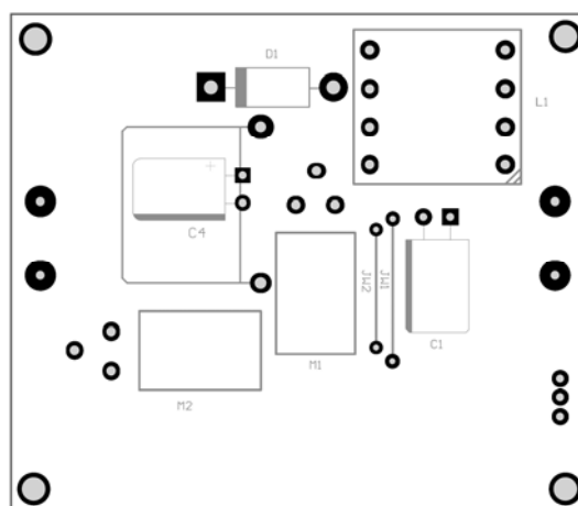
Figure 4—Bottom Layer
