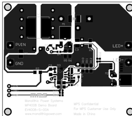
Figure 2—Top Layer
