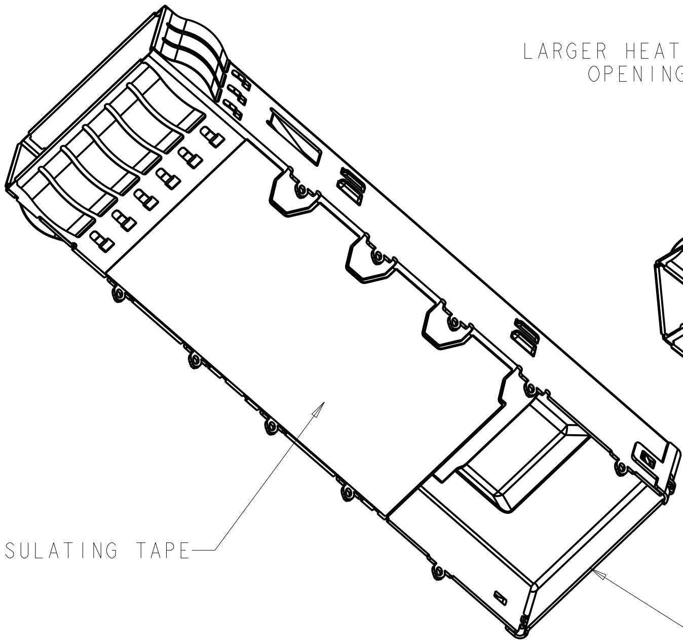
SCALE 3:1
