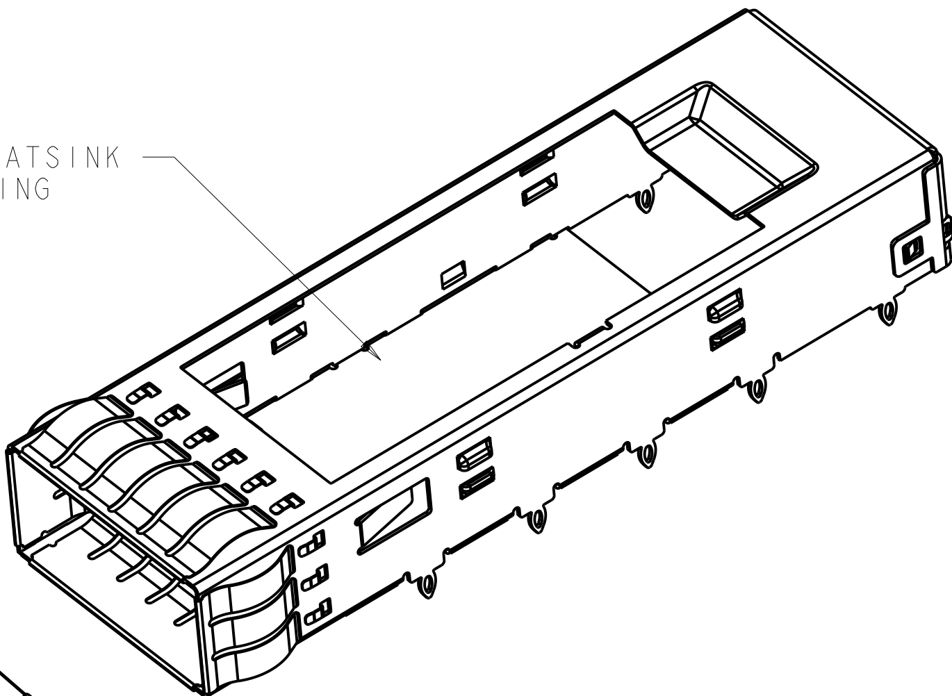
SCALE 3:1
