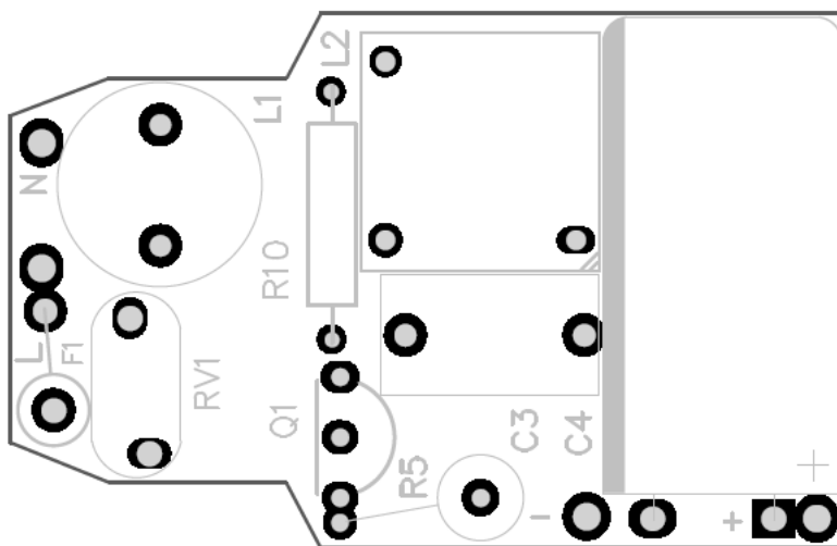
Figure 2—Top Layer
