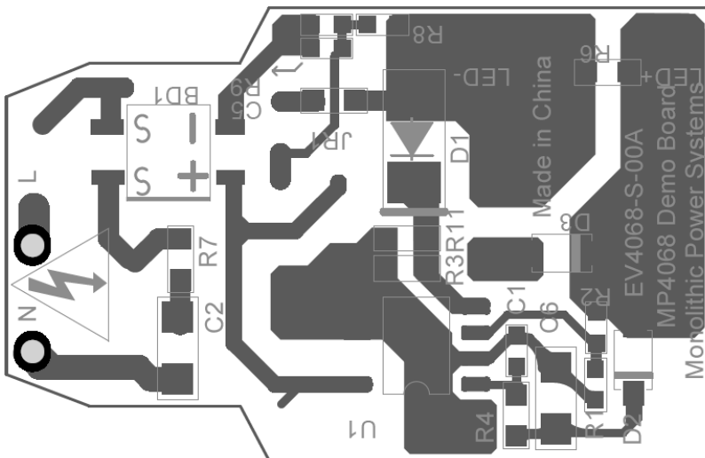
Figure 3—Bottom Layer
