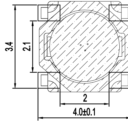
PCB板焊盘尺寸
