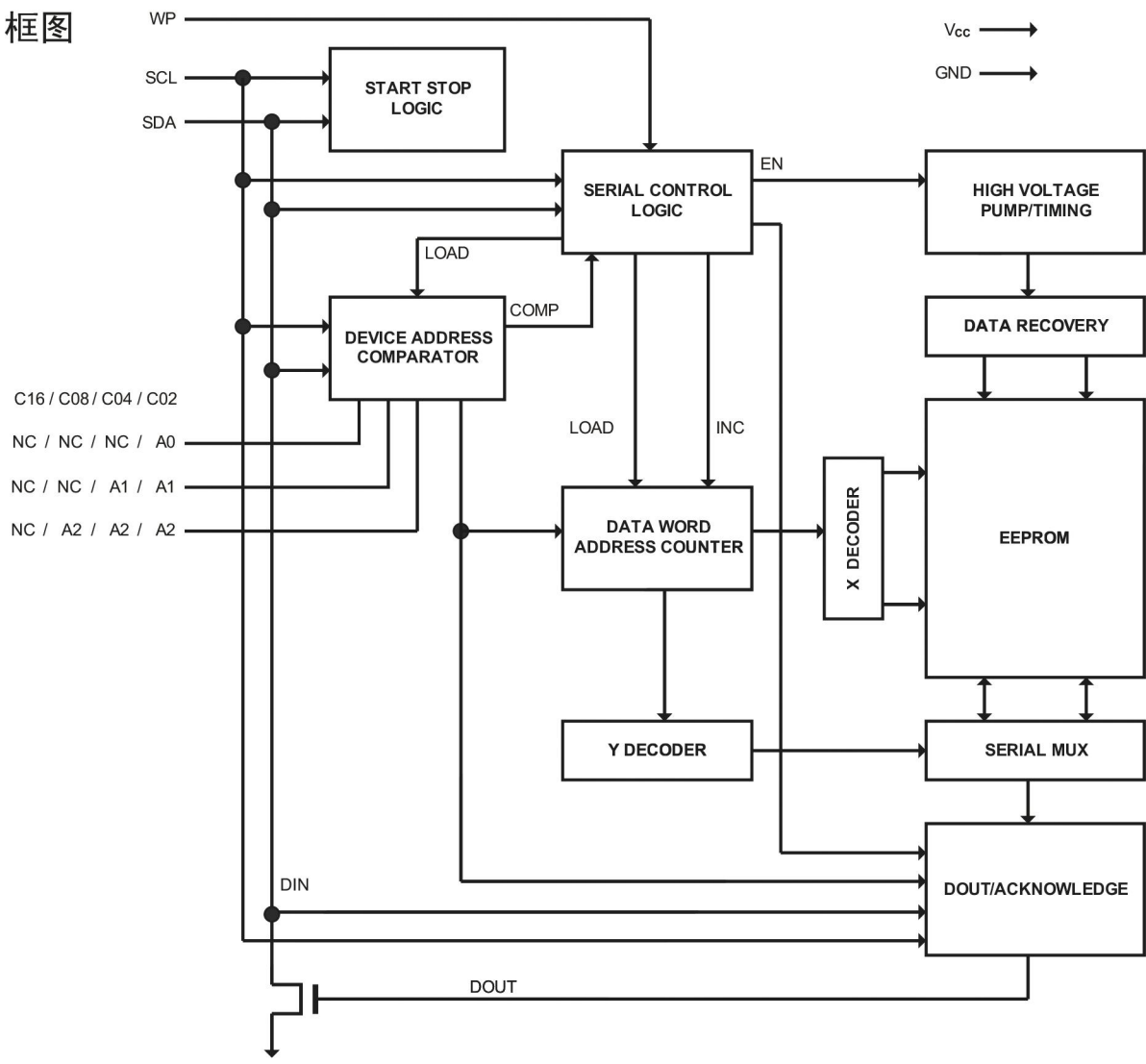
图1 框图
