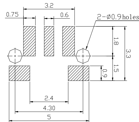
PCB. 焊接图
