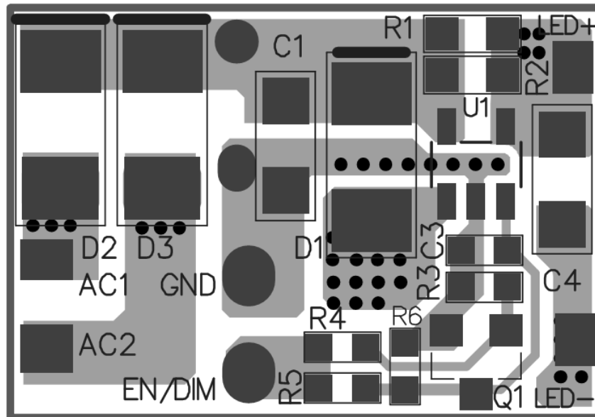
Figure 1—Top Layer
