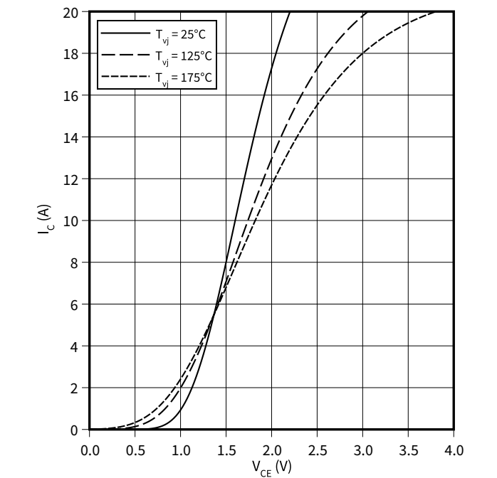
Ausgangskennlinie (typisch), IGBT, Brems-Chopper I_C = f(V_{CE}) V_{GE} = 15\text{ V}
