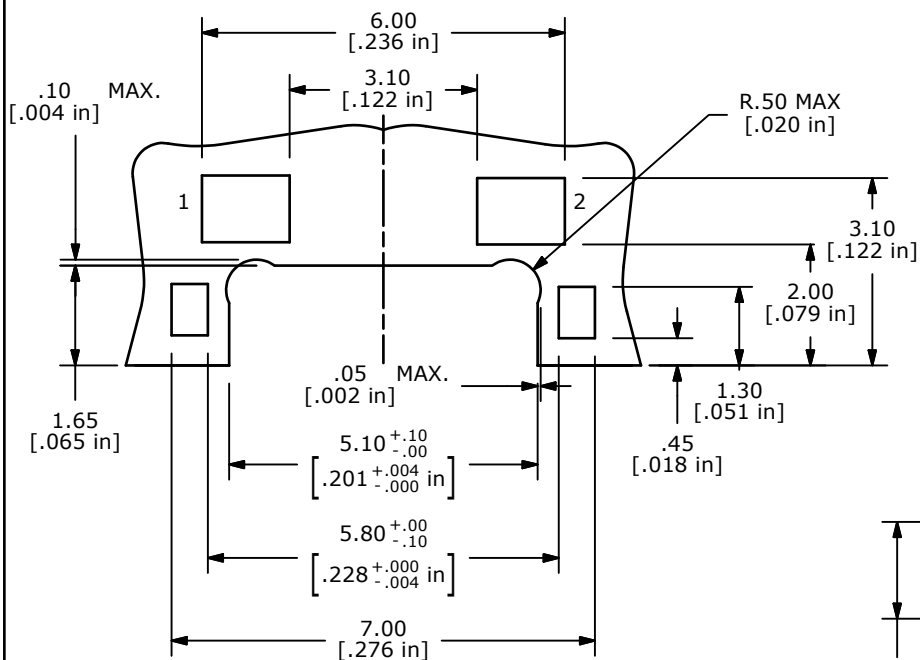
P.C.B. LAYOUT
