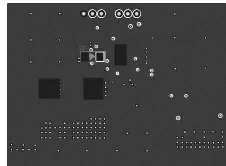
Bottom Layer
