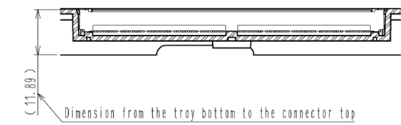
B-B(1:1)
