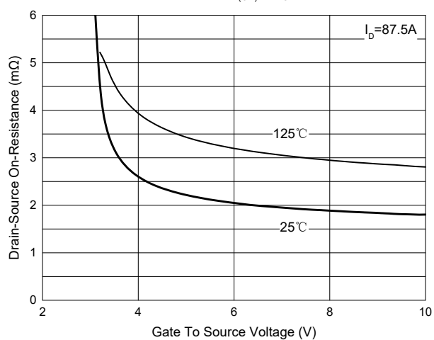
Fig. 3 - R_{DS(ON)} - V_{GS}
