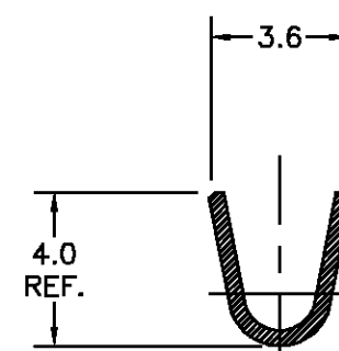
SECÇÃO A-A SECTION A-A
