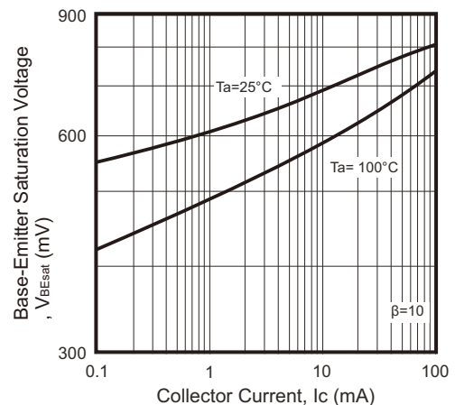
Fig.4 - V_{BEsat} - I_C
